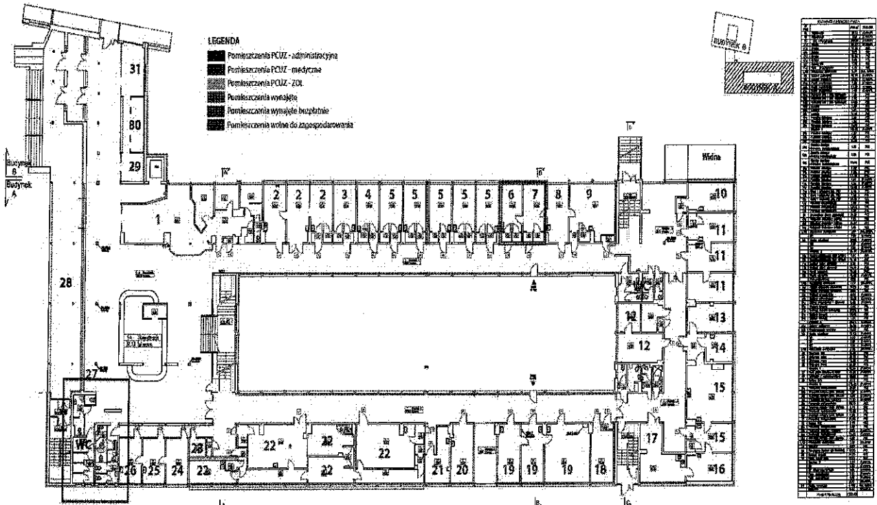
RZUT PARTERU 1:100
